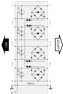
G : Eclateur à gaz tripolaire
